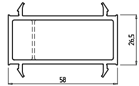
Соединительный профиль 26,5 мм (с форкамерой) армирующий профиль: Арт. № 604 Арт. № 157 Соединительный профиль 26,5 мм (без форкамеры) армирующий профиль: Арт. № 205 Арт. № 158
