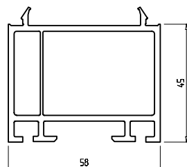
Расширитель 45 мм армирующий профиль: Арт. № 219 Арт. № 545
