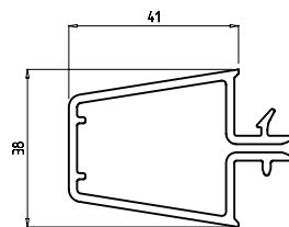
Крепежный кожух-крышка армирующий профиль: Арт. № 209 Арт. № 153
