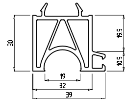
Стыковочный профиль к подоконнику 30 мм (к Арт. № MST.U, MST.S) Арт. № 346F
