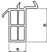
Соединительный профиль 35 мм Арт. № 143
