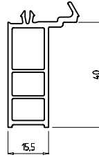
Универсальный соединитель 40 мм Арт. № 140
