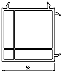
Угловой профиль 90° армирующий профиль: Арт. № 655 Арт. № 455
