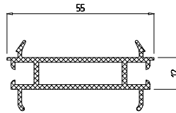
Алюминиевый соединитель Арт. № 180
