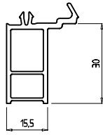
Универсальный соединитель 30 мм Арт. № 142
