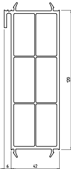
Соединитель/ расширитель 120 мм строит. глубина 42 мм Арт. № 347
