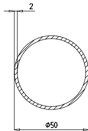
Армирующий профиль Арт. № 640
