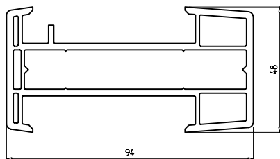
Н-образный соединитель армирующий профиль: Арт. № 208 монтажные анкера: Арт. № AR 152, AL 152, AI 152 Арт. № 152
