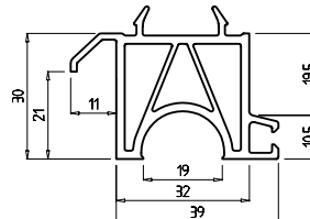
Стыковочный профиль к подоконнику 30 мм (к Арт. № MST.U, MST.S) Арт. № 346
