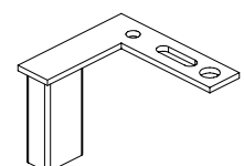
Крепежный анкер (к Арт. № 209) Арт. № A 153
