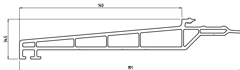
Подоконник , 140 мм выступ (к Арт. № 108, 109, 309, 308, 308-20) Арт. № FB 140
