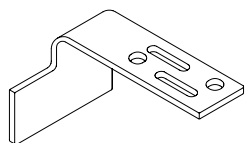
Крепежный анкер правый (к Арт. № 152) Арт. № AR 152
