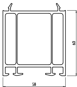
Расширитель 60 мм армирующий профиль: Арт. № 219 Арт. № 546
