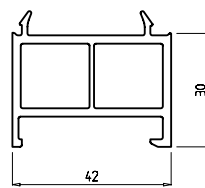
Расширитель 30 мм строит. глубина 42 мм Арт. № 548 Арт. № 548R
