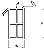
Соединительный профиль 35 мм Арт. № 143
