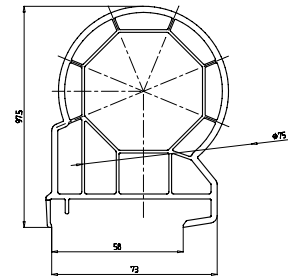
Угловой соединитель Арт. № 540
