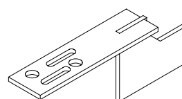
Крепежный анкер изнутри (к Арт. № 152) Арт. № AI 152
