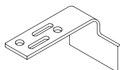
Крепежный анкер левый (к Арт. № 152) Арт. № AL 152
