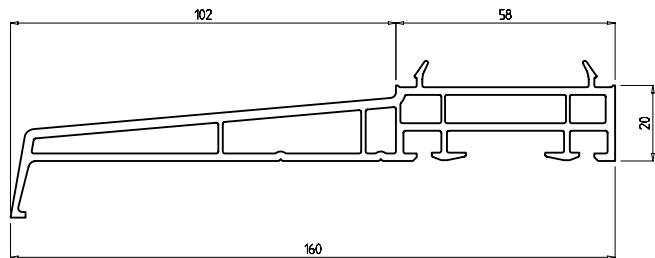
Подоконник 160 мм Арт. № FB 102
