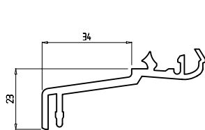
Козырек-отлив для подоконника, 21/34 мм выступ Арт. № FB 34
