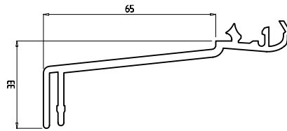
Козырек-отлив для подоконника, 52/65 мм выступ Арт. № FB 65
