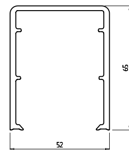
Пиластровый профиль армирующий профиль Арт. № 614 Арт. № 154
