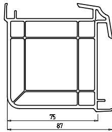
Угловой профиль 90° армирующий профиль: Арт. № 655 Арт. № 155
