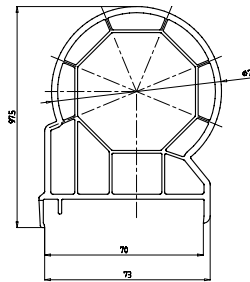
Угловой соединитель Арт. № 340
