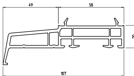
Подоконник 107 мм Арт. № FB 49
