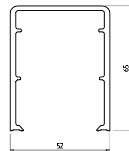
Пилястровый профиль армирующий профиль Арт. № 614 Арт. № 154
