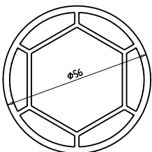
Труба из ПВХ 56 мм Армирующий профиль: труба 33,7 мм Арт. № 643 Арт. № 543
