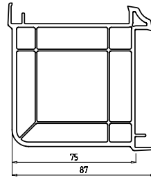
Угловой профиль 90° армирующий профиль: Арт. № 655 Арт. № 355
