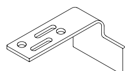
Крепежный анкер левый (к Арт. № 152) Арт. № AL 152
