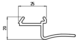
Прокладочный профиль для облицовочных плит Арт. № 552
