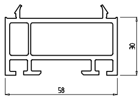
Расширитель 30 мм армирующий профиль: Арт. № 602 Арт. № 144
