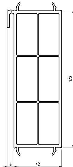
Соединитель/ расширитель 120 мм строит. глубина 42 мм Арт. № 347
