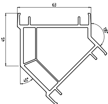
Угловой профиль 135° армирующий профиль: Арт. № 656 Арт. № 156
