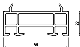
Расширитель 22 мм (для вентиляционного клапана "Климабокс") Арт. № 741
