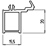
Универсальный соединитель 20 мм Арт. № 139
