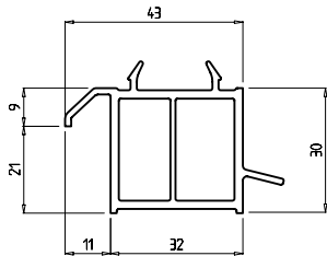
Соединительный профиль 30 мм x 32 мм Арт. № 343
