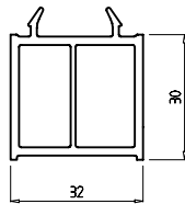
Соединительный профиль 30 мм Арт. № 343R
