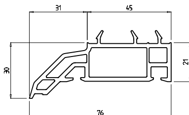
Подоконник 76 мм, армирующий профиль: Арт. № 606 Арт. № FB 31
