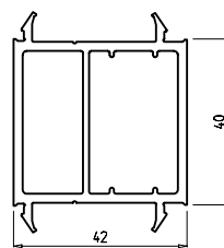
Соединитель/расширитель 40 мм строит. глубина 42 мм армирующий профиль: Арт. № 203 Арт. № 549
