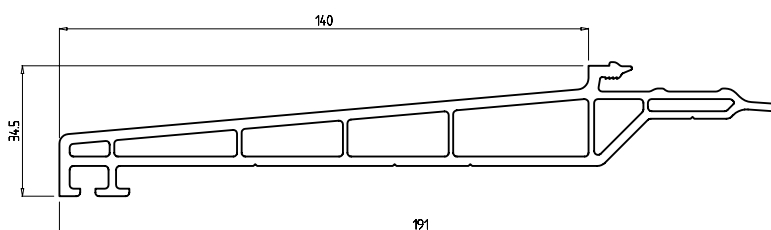
Подоконник , 140 мм выступ (к Арт. № 108, 109, 309, 308, 308-20) Арт. № FB 140
