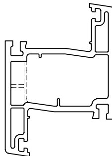
Профиль с чередованием упора 82 мм Арт. № 539 (без форкамеры) Арт. № 538
