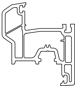
Реставрационная створка «антик» 77 мм Арт. № 315
