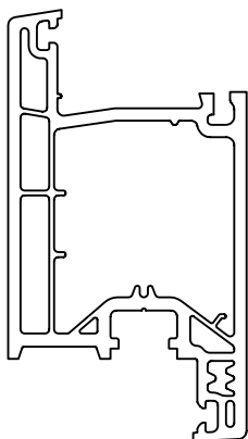
Створка 105 мм (в разных плоскостях с рамой) Арт. № 119
