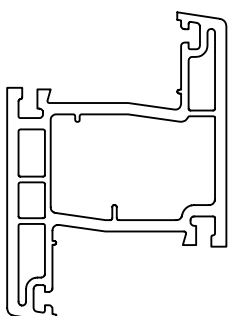
Профиль 82 мм с чередованием упора Арт. № 539
