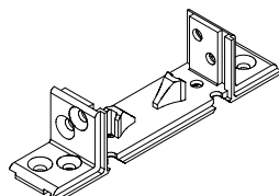
Соединитель импоста (к Арт. № 715) Арт. № V 715
