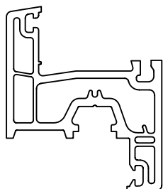
Створка 69 мм (в разных плоскостях с рамой) Арт. № 117
