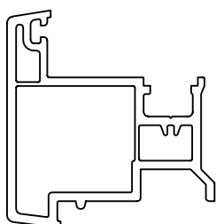
Штульп -/ створка средне-подвесная 65 мм (без форкамеры) Арт. № 734S
