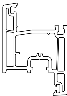
Створка 82 мм (в разных плоскостях с рамой) Арт. № 318
