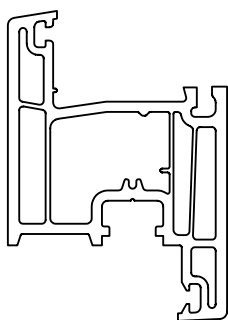
Створка 77 мм (четырёхкамерная) (в разных плоскостях с рамой) Арт. № . 314
