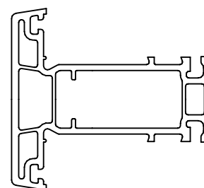
Переплет-поперечина створки 68 мм (в одной плоскости с рамой) Арт. № SP 135
