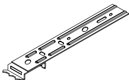
Монтажный анкер (к Art. № 132, 532, 539, 538) Art. № 620
