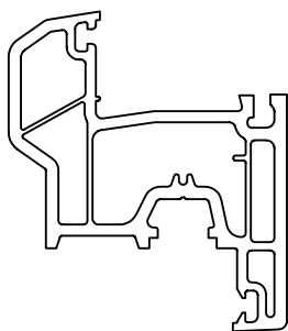
Реставрационная створка «антик» Арт. № . 315
