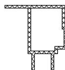
Распорочный профиль из алюминия для неподвижной части (к Art. № 769) Art. № 787
