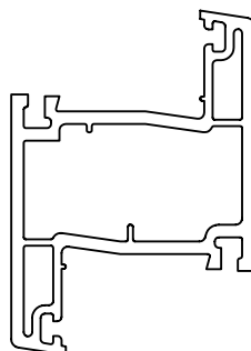
Профиль 82 мм с чередованием упора( без форкамеры) Арт. № 538
