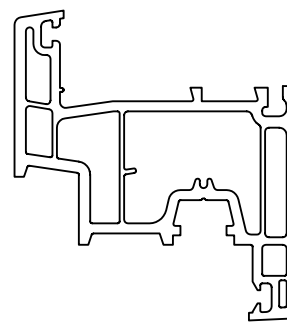
Створка 82 мм (в одной плоскости с рамой) Арт. № 316
