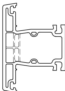
Импост 82 мм Арт. № 132 (без форкамеры) Арт. № 532
