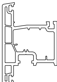
Т-образная створка 87 мм (в разных плоскостях с рамой) Арт. № 519
