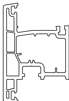
T - образная створка 87 мм (в разных плоскостях с рамой) Арт. № 519
