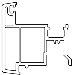
Штульп/ створка средне- подвесная 65 мм Арт. № 734
