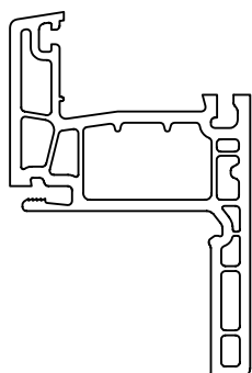
Реставрационная рама 88 мм Арт. № 109
