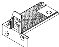
Соединитель порога для порожка Art. № 788 к раме Art. № 107 Art. № SH 107
