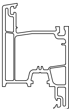
Створка 92 мм (в разных плоскостях с рамой) Арт. № 713
