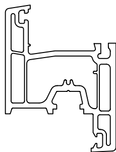
Створка 77 мм (в разных плоскостях с рамой) Арт. № 317
