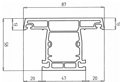
Импост Арт. № 337
