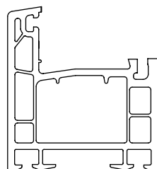
Рама Арт. № 807
